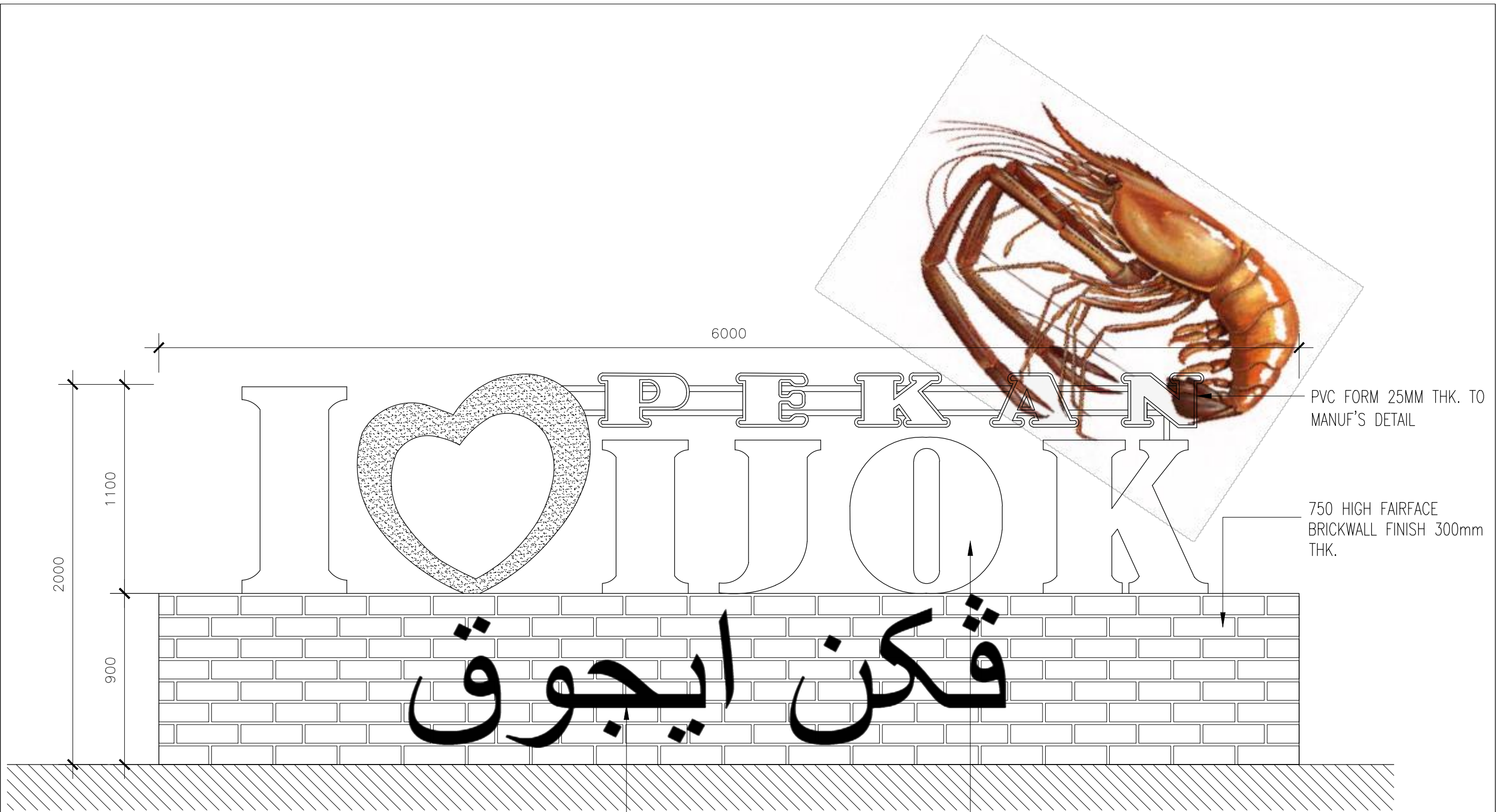
PANDANGAN HADAPAN SKALA 1:20
