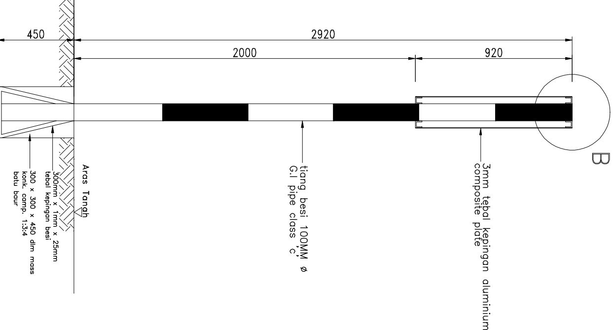
KERATAN A-A (SKALA 1 : 10)
