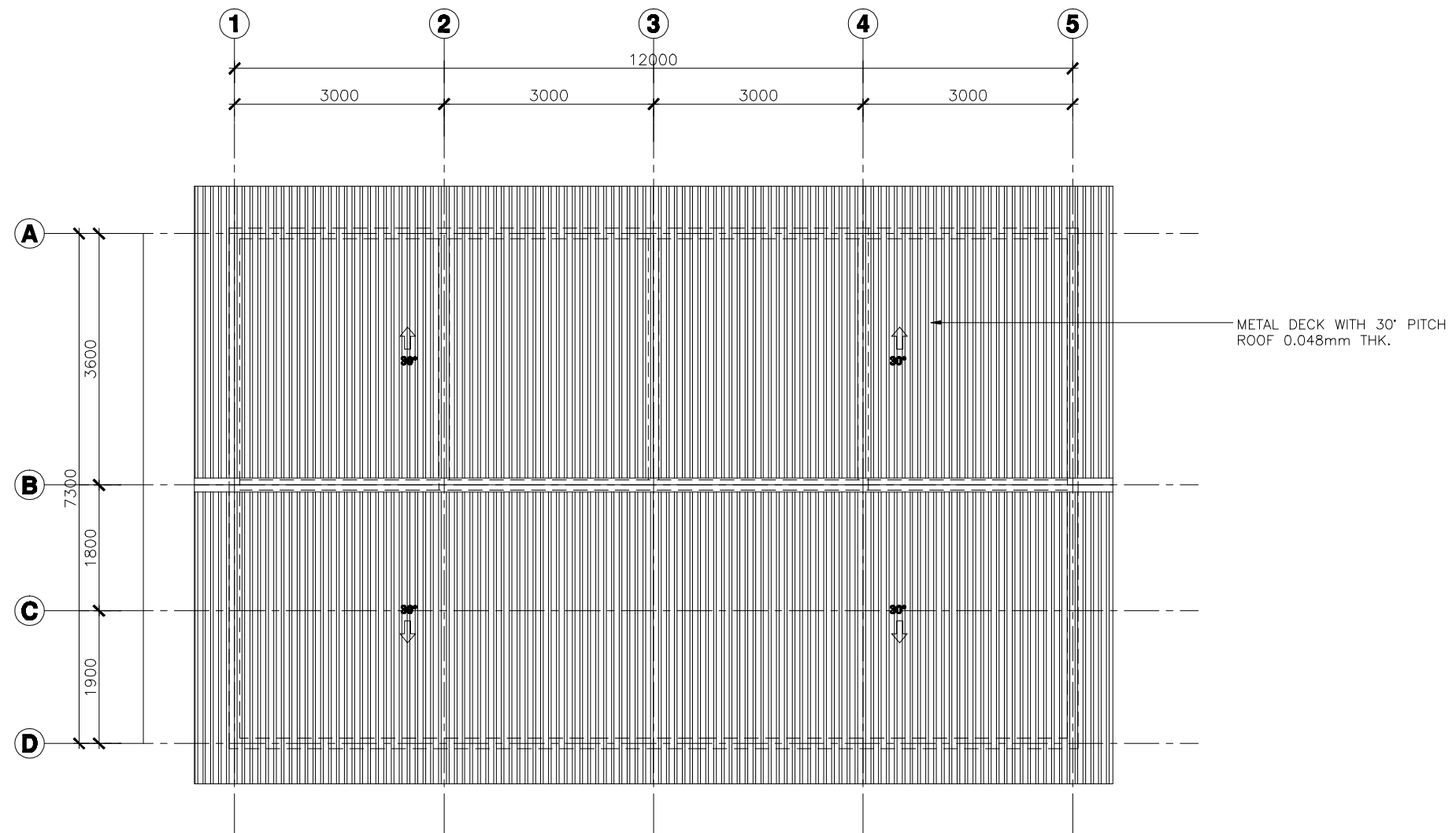
PELAN BUMBUNG SKALA 1:75
