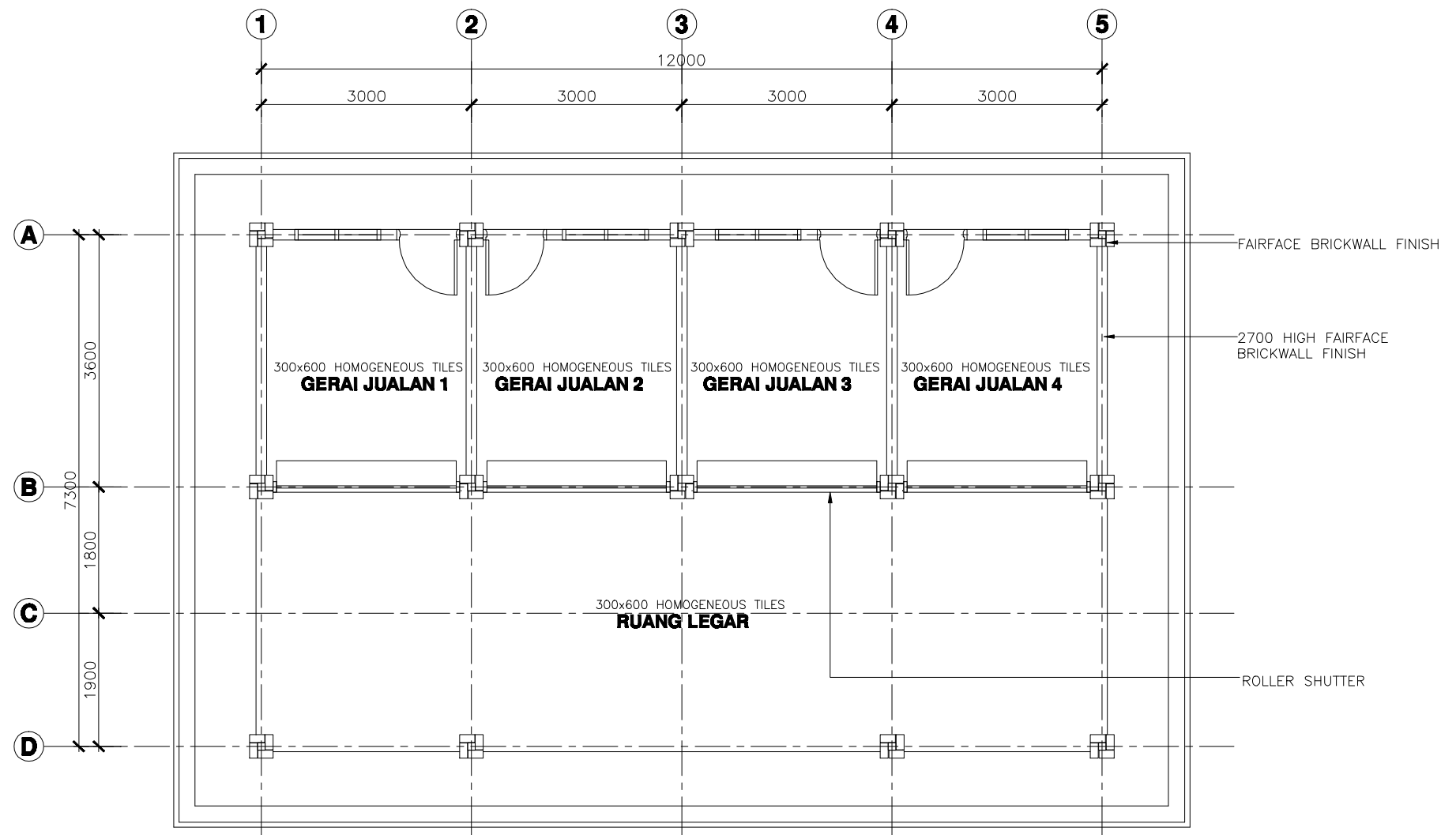
PELAN LANTAI SKALA 1:75
